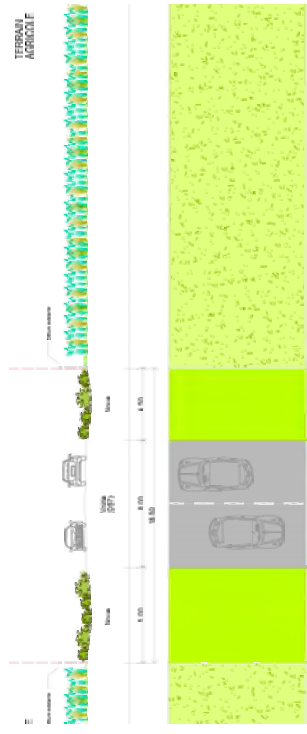
Profil existantEG
