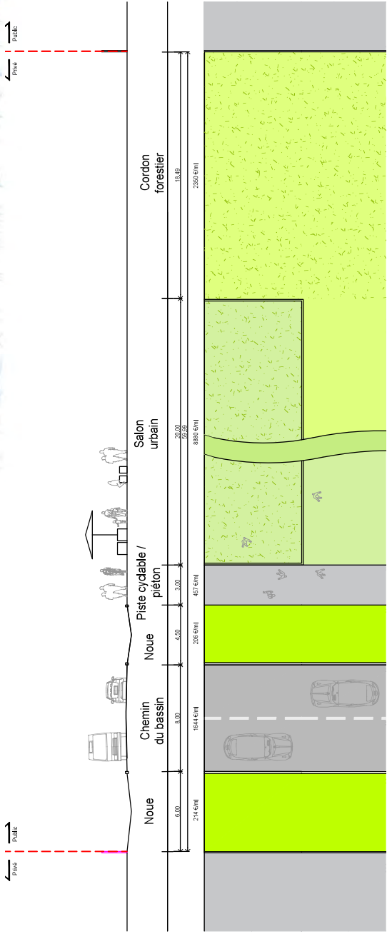
Profil sur le corridor actif
